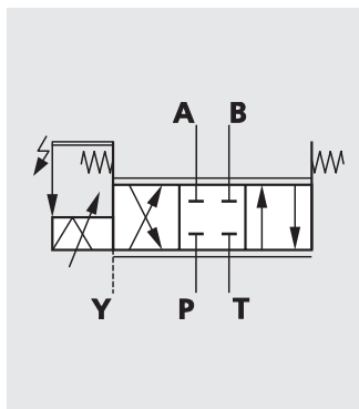
四通阀规格 弹簧对中
